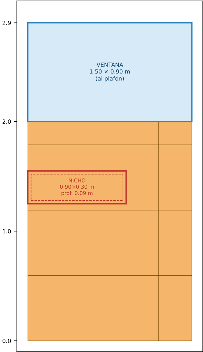
Regadera 2 (P.A.) muro de fondo 1.50 × 2.90 m 3 caras – ventana = 9.96 m²
